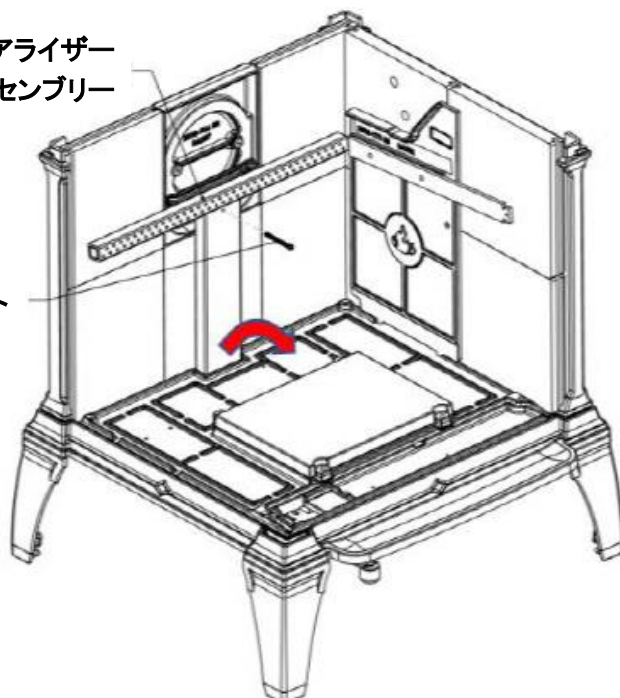
ボルト
