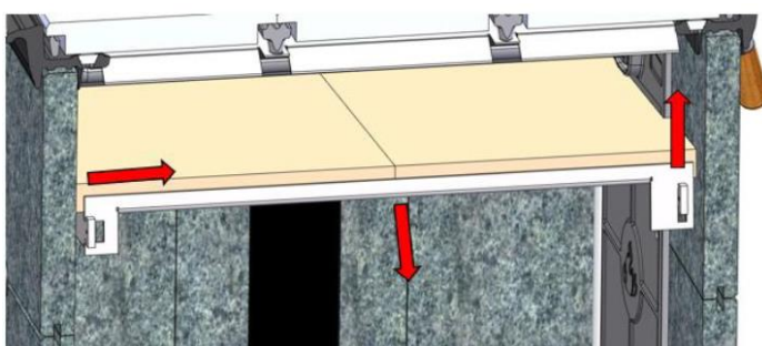
A) バッフル・プロテクターを外します
