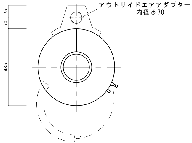
平面図
